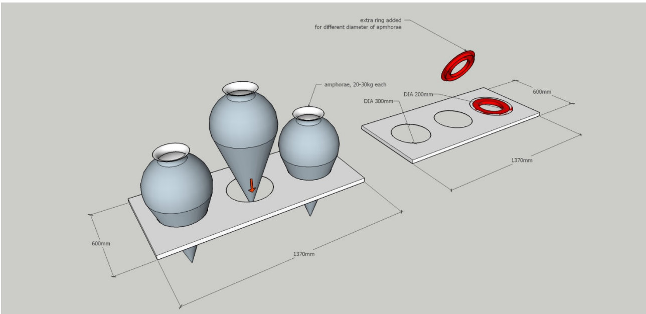
Σχέδιο 2. Ειδική κατασκευή αποθηκευτικών επιπέδων (συστοιχίες τύπου 3) (ενδεικτικό σχέδιο).
